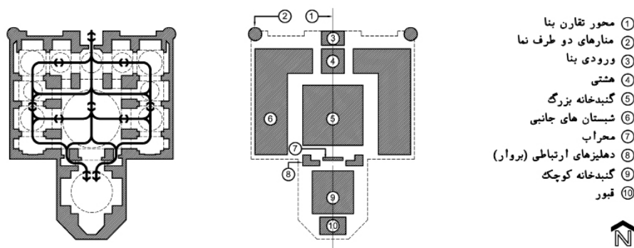
تصویر ۴: روابط عاصر و ریز فضاهای مسجد کبود
