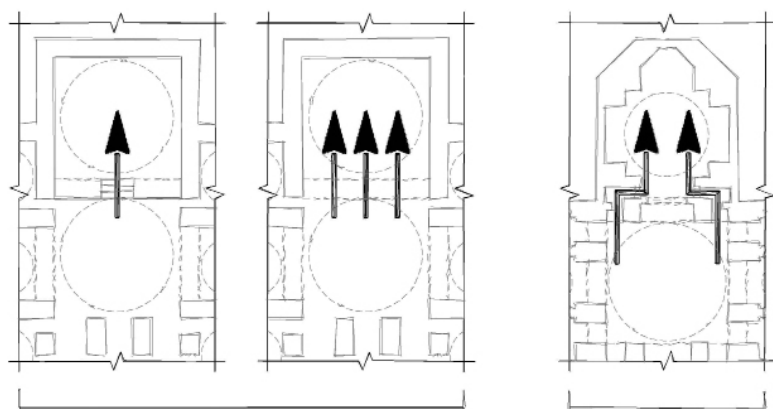
تصویر ۱۴: مقایسه روابط بین دو گنبدخانه در نمونه‌های منطقه آناتولی و مسجد کبود
